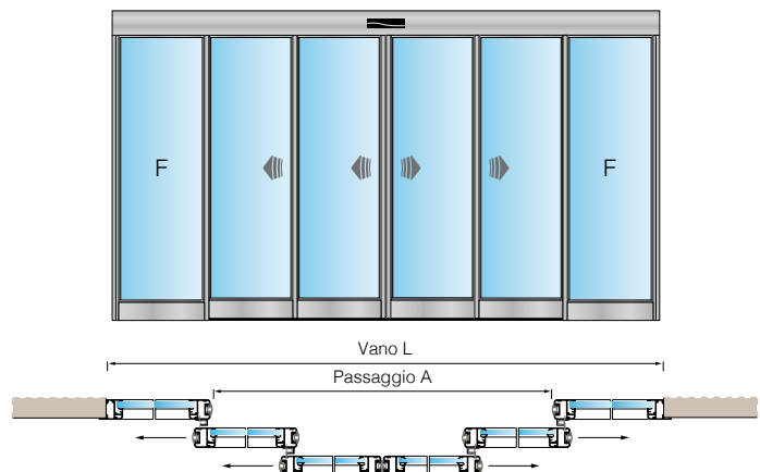
TSA BILATERAL 6 ANTE (4 MOBILI + 2 FISSE)
