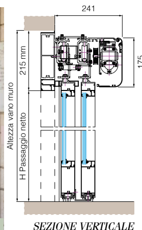
SEZIONE VERTICALE
