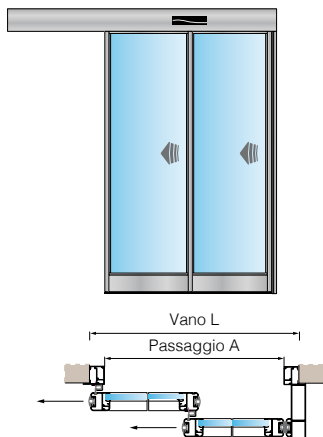
TSA 2+1 ante scorrevoli in chiusura
