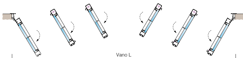
TSA TOS BILATERAL (4 ante mobili + 2 semifisse) per uscita di sicurezza
