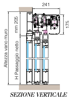
SEZIONE VERTICALE
