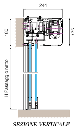
SEZIONE VERTICALE
