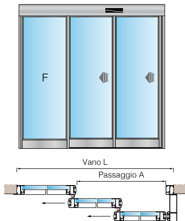
Profilati da 20 mm
