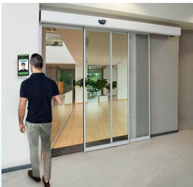
Termocamera PONZI RFT installata su parete. Collegata a porta d'ingresso automatica singola.
